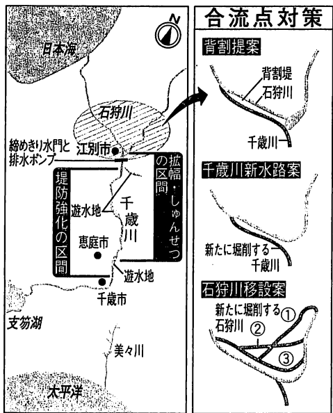
図。道がまとめた千歳川の総合治水対策
