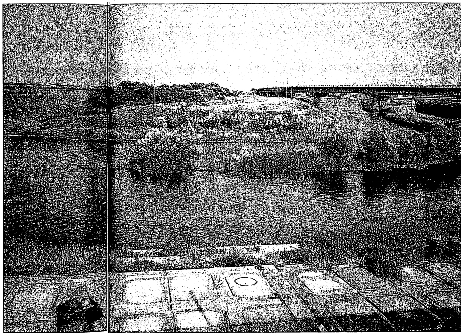
千歳川(右手)と石狩川との合流点。ここに背割堤を造ったり、左手の石狩川を北側に移設する案などが今後の検討課題になっている。
